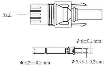
Fig. 3.1 Conector macho DC
