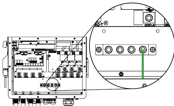
Ligação à terra (fios de cobre)
