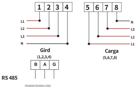
Fig. 7.3 Medidor Eastron
