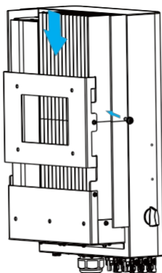
Fig. 4.6 Instalação do inversor
