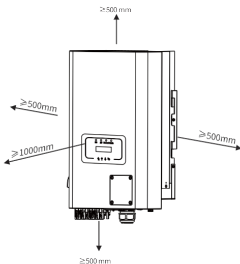
Fig. 4.3 Espaço de instalação
