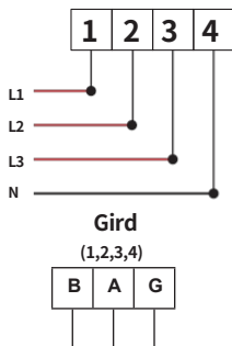
Fig. 7.1 Medidor Eastron
