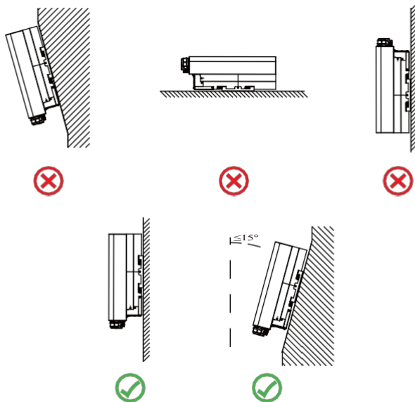
Fig. 4.2 Ângulo de instalação
