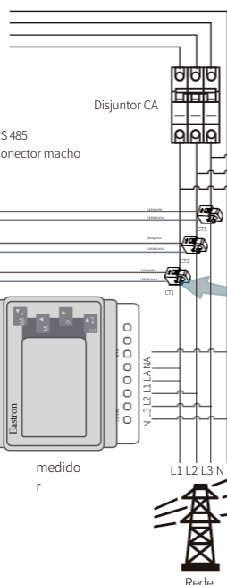
Fig. 7.6 Diagrama de conexão do medidor Eastron
