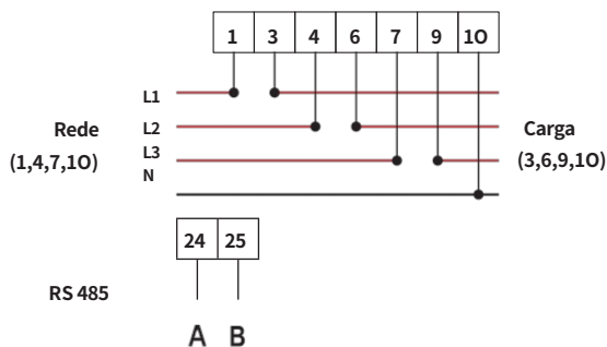
Fig. 7.11 Medidor CHNT
