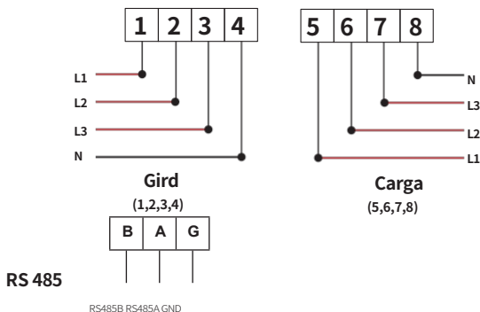
Fig. 7.18 Medidor Eastron
