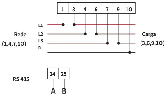
Fig. 7.28 Medidor CHNT
