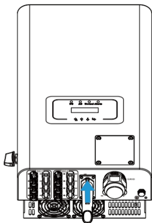
Fig. 5.13 Diagrama de instalação do registador de dados
