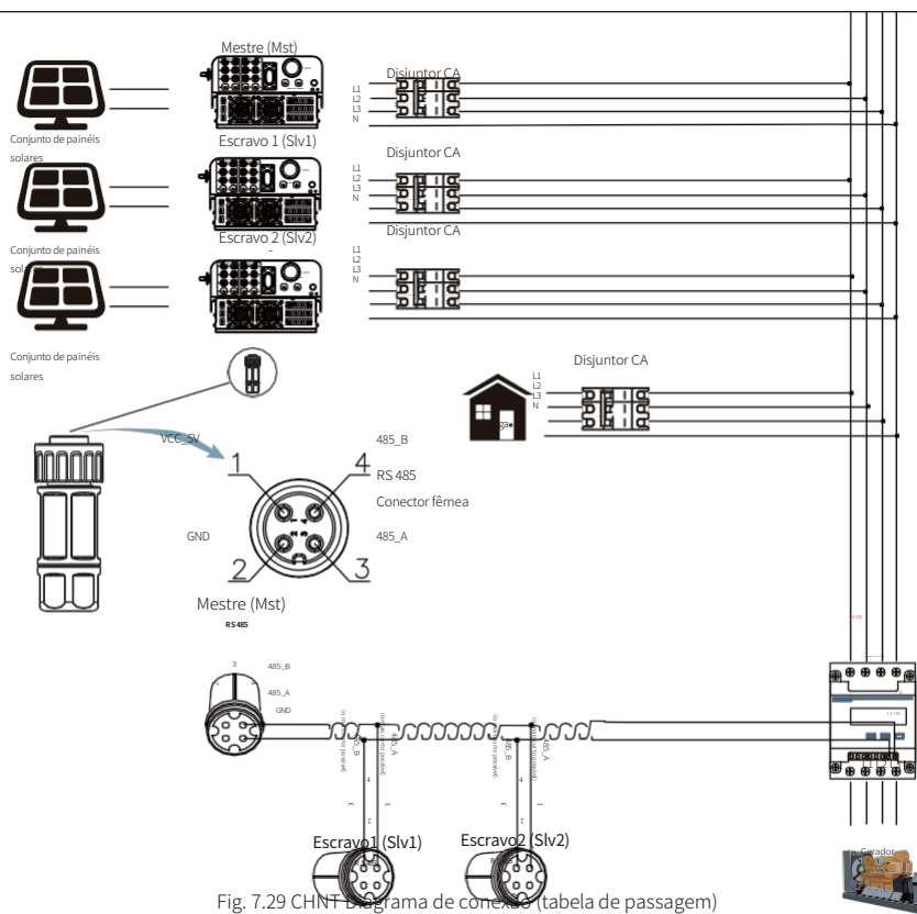
Fig. 7.29 CHNT Diagrama de conexão (tabela de passagem)
