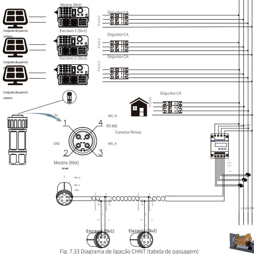
Fig. 7.33 Diagrama de ligação CHNT (tabela de passagem)
