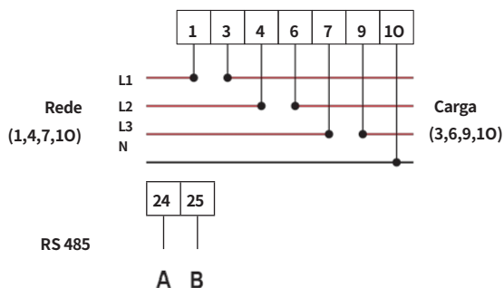
Fig. 7.9 Medidor CHNT
