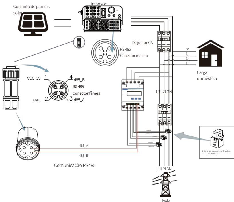
Fig. 7.14 Diagrama de ligação do medidor CHNT
