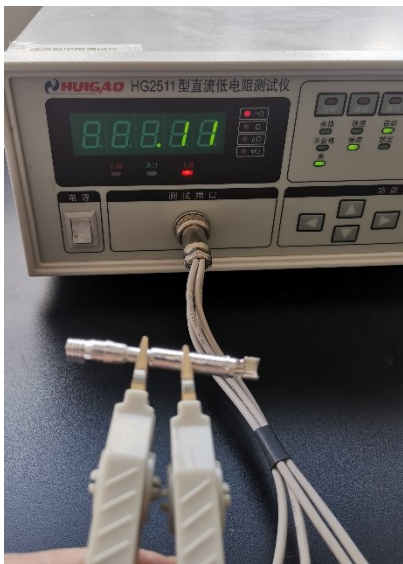
图片 5 插套 & MC4 插针 socket & MC4 pin
