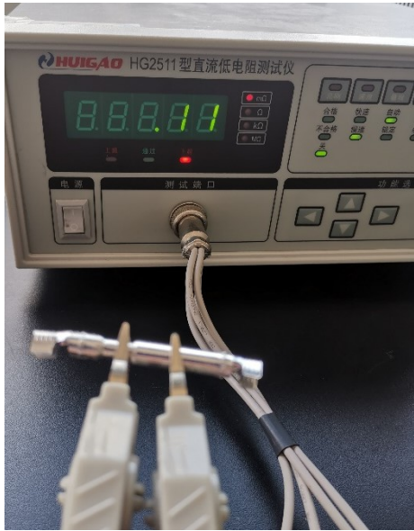
图片 3 插套 & T4 插针 socket & T4 pin
