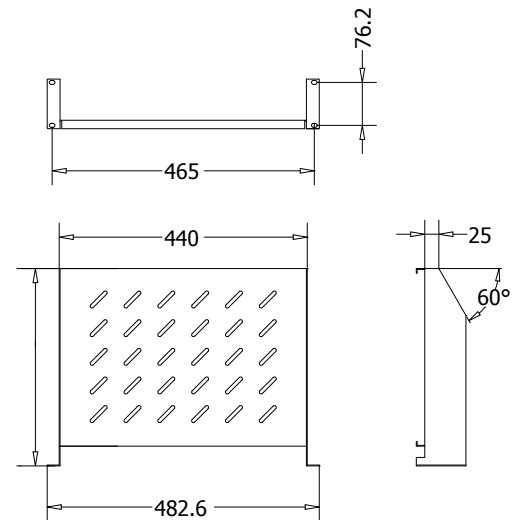
Bandeja 19" negra
