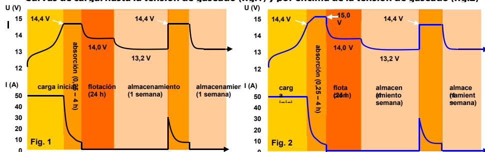
Curvas de carga: hasta la tensión de gaseado (fig.1) y por encima de la tensión de gaseado (fig.2)
